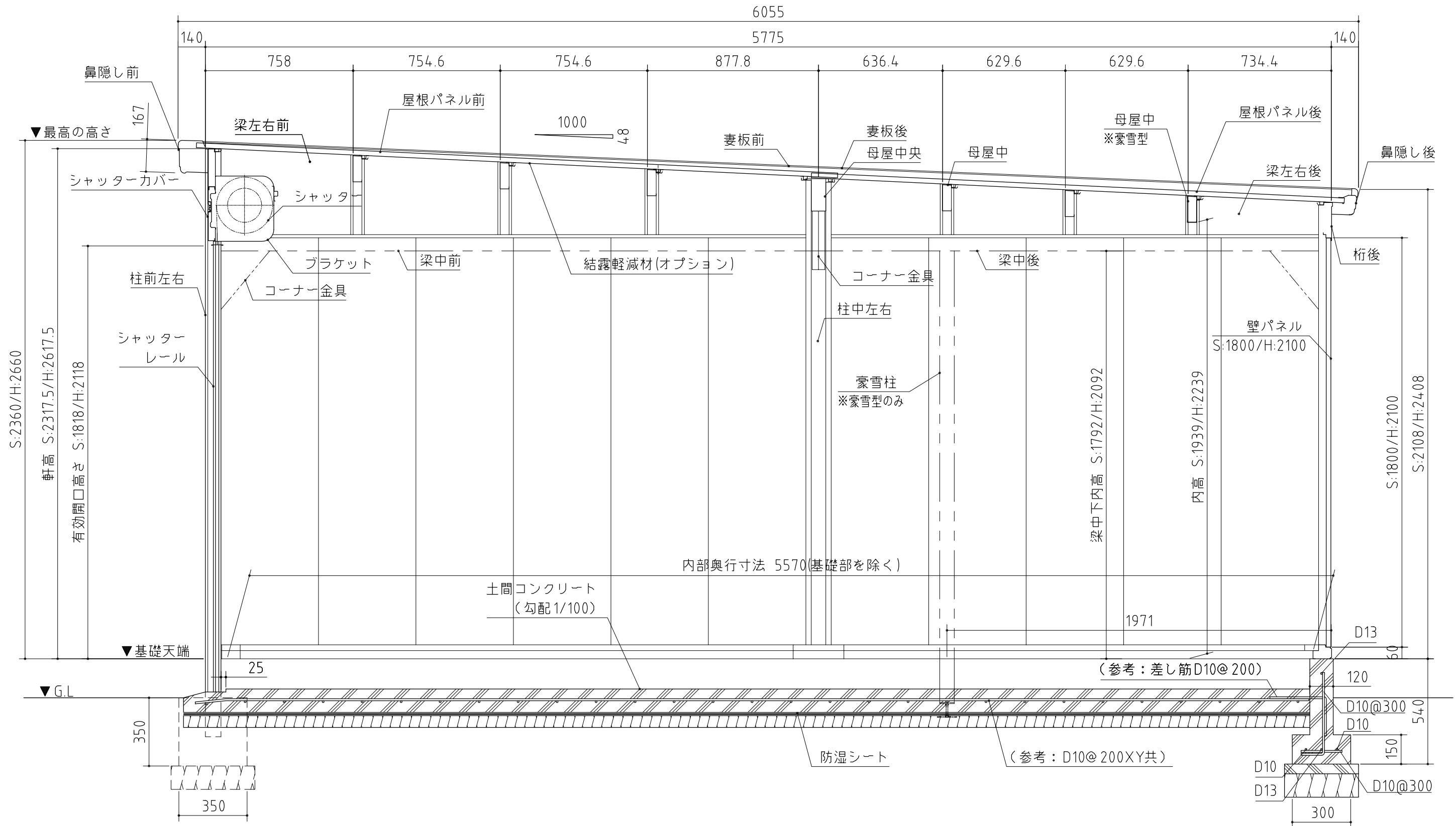
断面図(側面) <縮尺> S=1/20 ~一般型・豪雪型~ 機種名 GRN- 2657S・SL・H・HL、3157S・SL・H・HL 3657S・SL・H・HL
